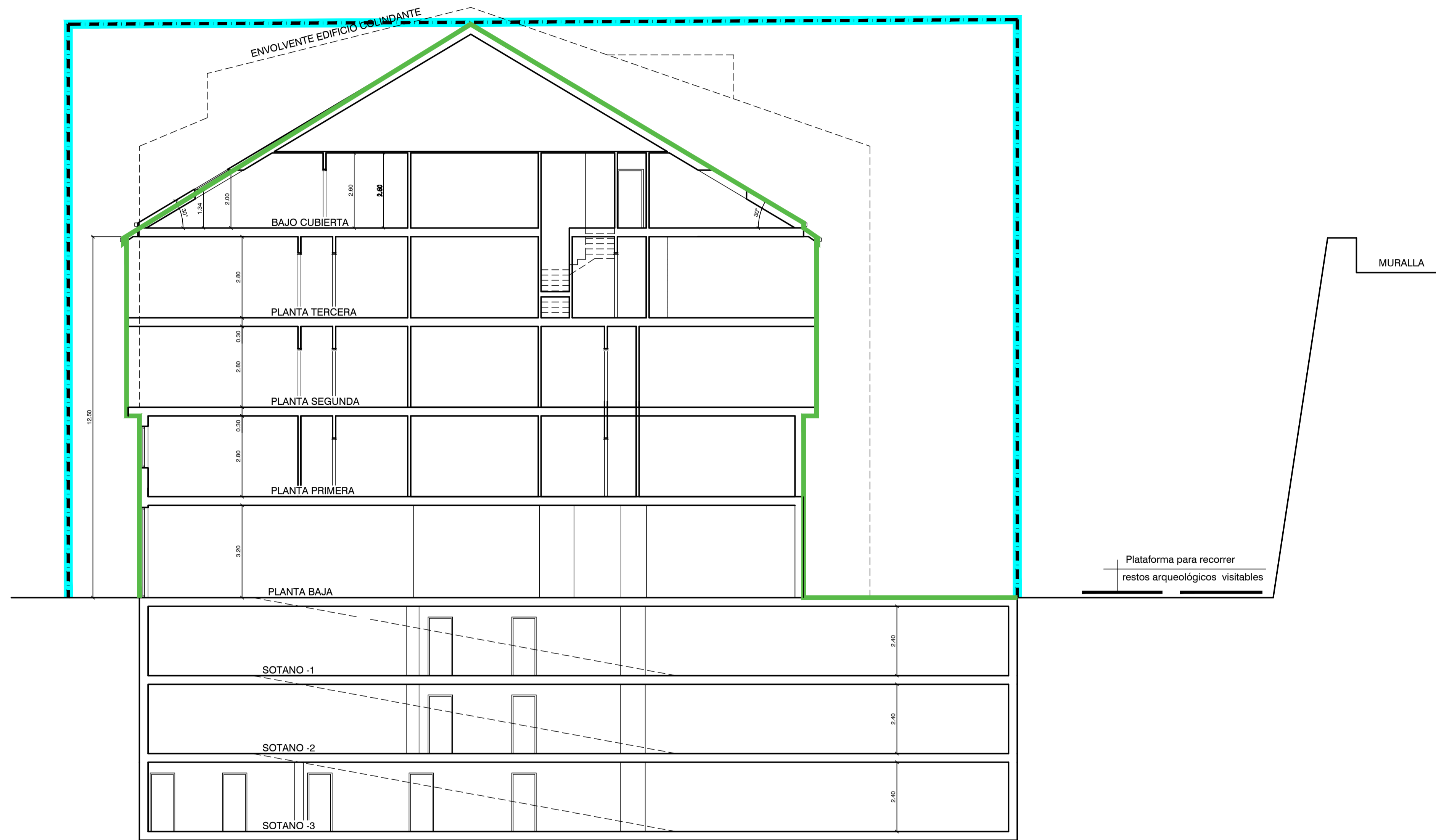
SECCION AB
