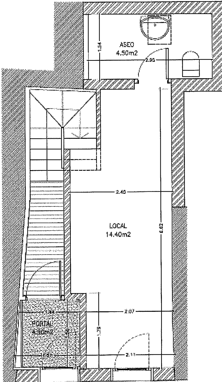
PLANTA BAJA
